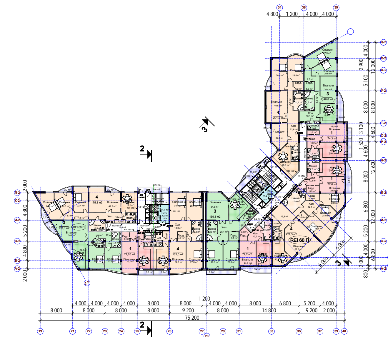
ПЛАН ТИПОВОГО ЖИТЛОВОГО ПОВЕРХУ
